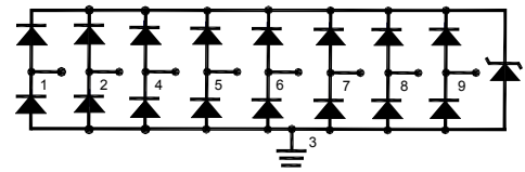
1. I/O 2. I/O 3. GND 4. I/O 5. I/O 6. I/O 7. I/O 8. I/O 9. I/O
