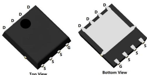
PDFN5*6-8L
